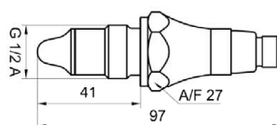
LBFS-xxAxx.x G 1/2 A DIN 3852-E (BCID: G51)
