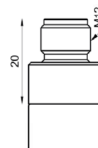
LBFS-x3xxx.x Steckverbindung M12-A, 4-Pin, Edelstahl (ohne LED)
