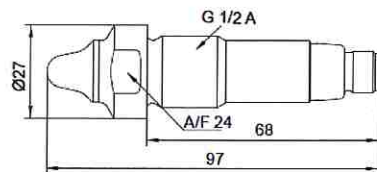
LBFS-xx5xx.x G 1/2 A ISO 228-1 für Innenmontage
