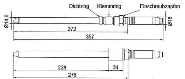
LBFS-xxLxx.x G 1/2 A hygienerecht, verschiebbarer Anschluss, Länge 250 mm
