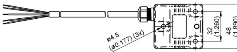
GIM500R - câble
