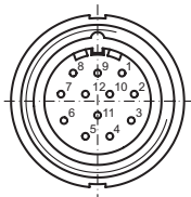
Connecteur M23, femelle, 12 points, rotation vers la gauche (CW)
